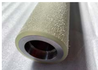
製鉄用 表面凹凸加工ロール
